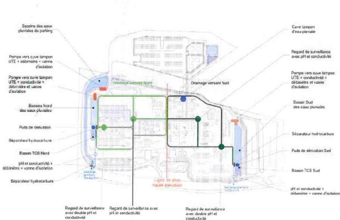
Figure 4: Gestion des eaux pluviales en phase d'exploitation - Usine
