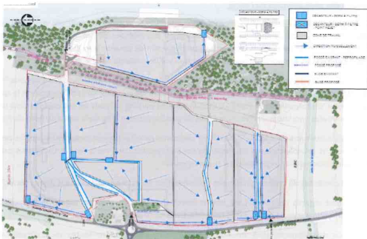
Figure 1: Schéma de gestion des eaux pluviales en phase travaux
