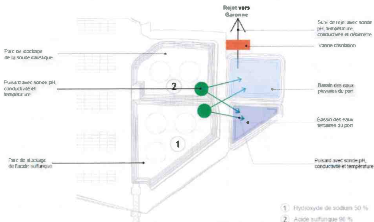
Figure 5: Gestion des eaux pluviales - Port
